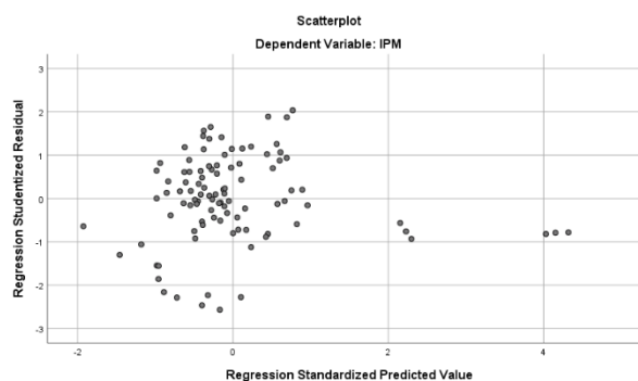
Gambar 1: Uji Heteroskedastisitas
