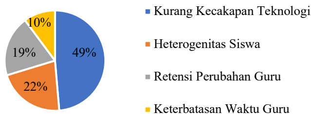
Gambar 3. Faktor Penghambat
