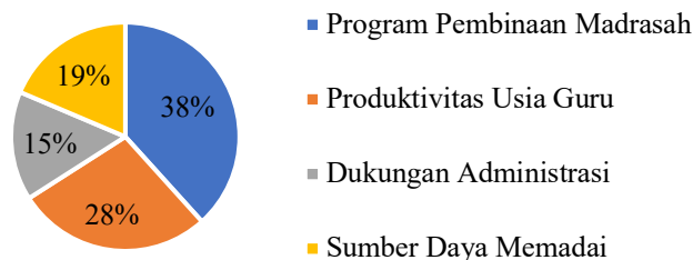
Gambar 2. Faktor Pendukung
