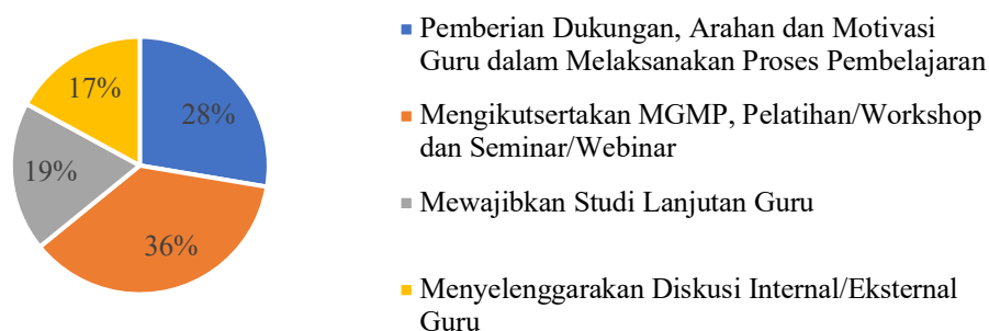
Gambar 1. Strategi Pembinaan
